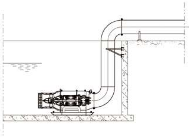
卧式安装示意图
