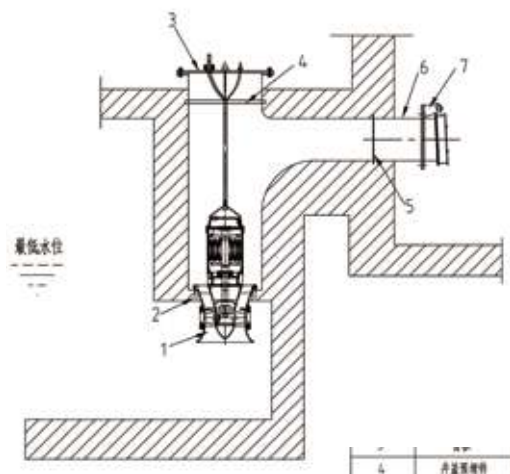
水泥井筒悬吊式安装示意图
