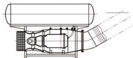
浮筒式安装示意图
