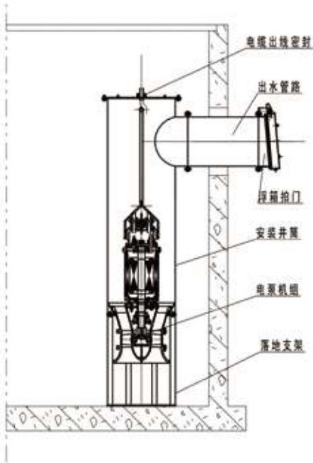
落地安装示意图
