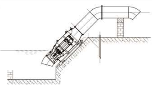
斜拉式安装示意图
