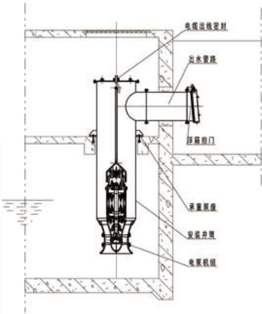
悬吊式安装示意图
