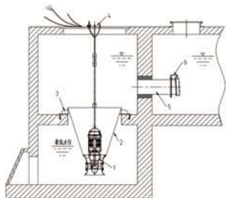
井筒敞开式安装示意图
