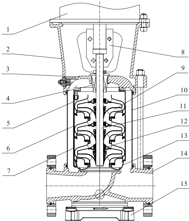
结构图LCS/LCA 32,45,64,90
